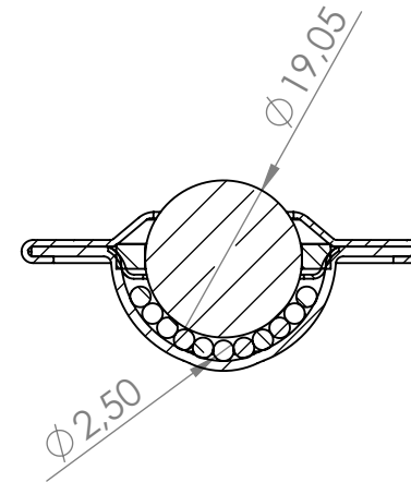
SCHNITT B-B
