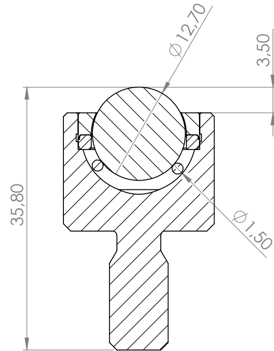
SCHNITT A-A
